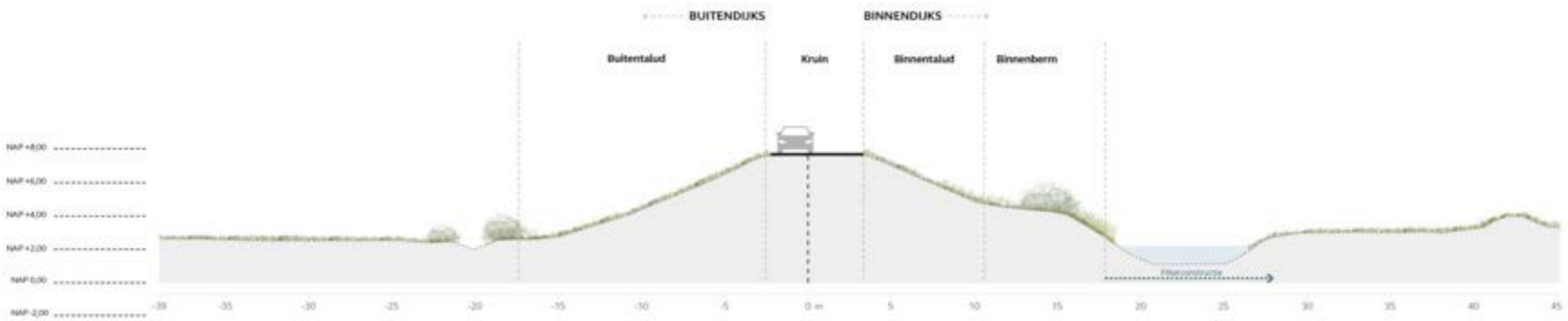
Dijkzone 2A – Vak 15+16a+17+18 – Alternatief 2 – Filterconstructie gracht
