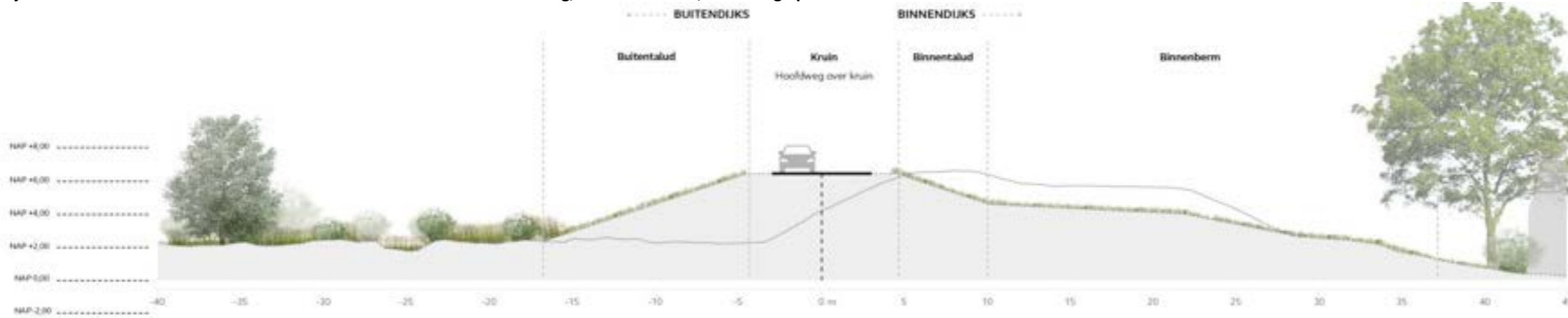
Dijkzone 11 – Vak 81+82+86a – Alternatief 2 – Buitenwaartse asverschuiving, kruin 9 m breed, hoofdweg op kruin
