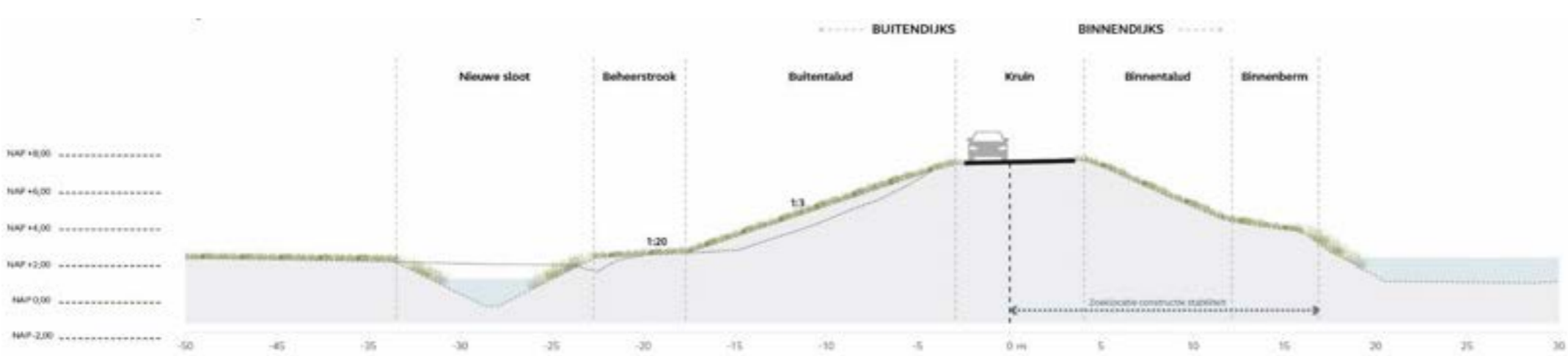
Dijkzone 2A – Vak 18 – Alternatief 1 – Stabiliteitsscherm
