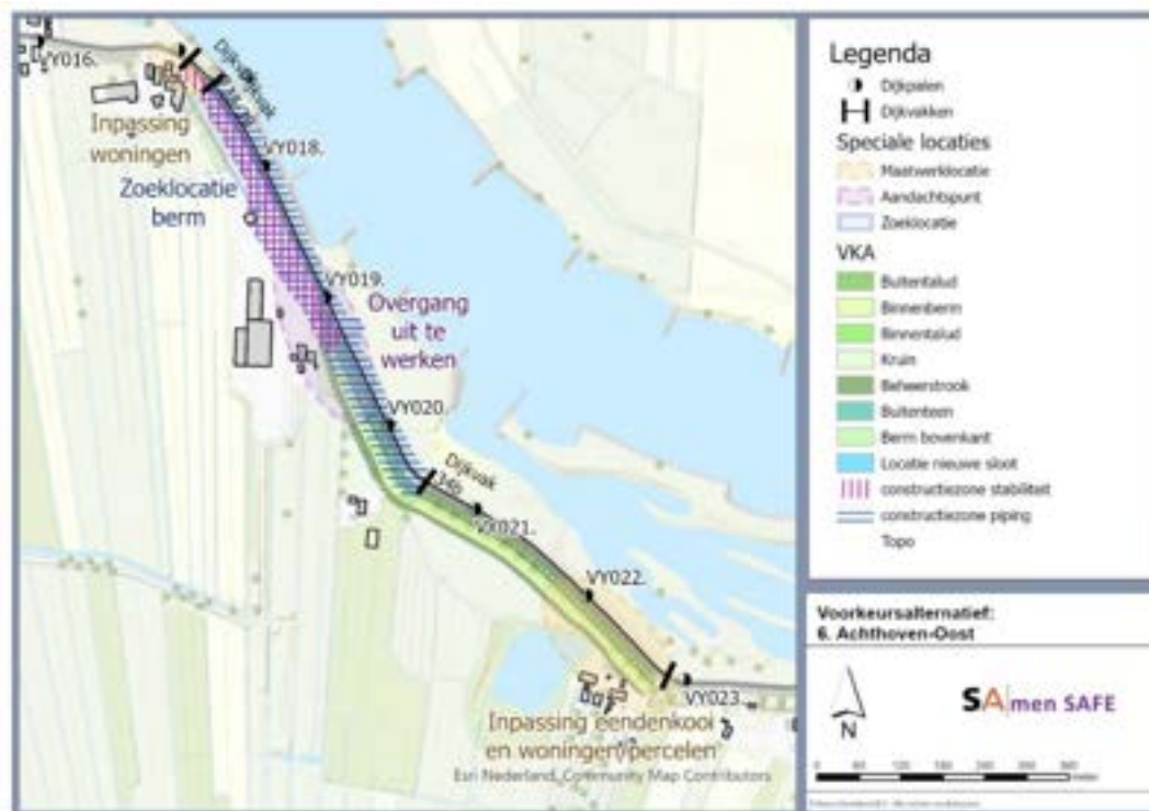
Figuur 9.1: Bovenaanzicht van het voorkeursalternatief bij dijkzone 6. NB pipingogave mist in het zuidoostelijke deel
