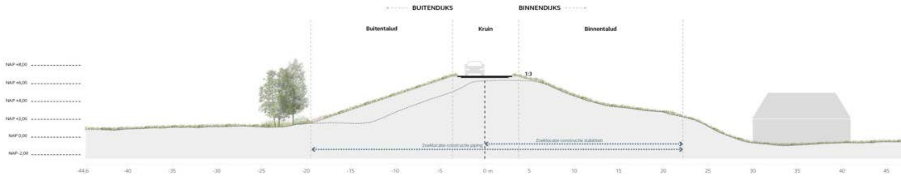
Dijkzone 10 – Vak 60 – Alternatief 2 – Buitenwaartse kruinophoging en constructie stabiliteit en piping
