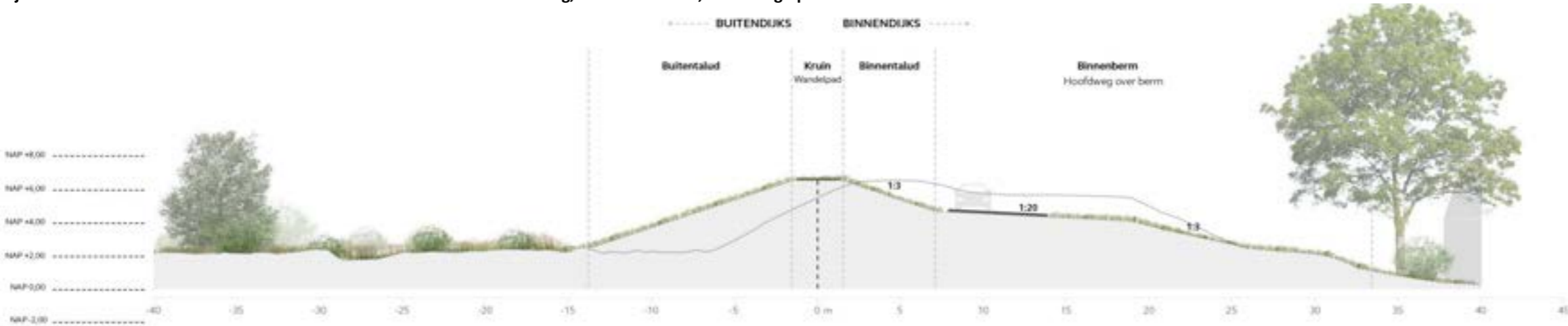
Dijkzone 11 – Vak 81+82+86a – Alternatief 3 – Buitenwaartse asverschuiving, kruin 3 m breed, hoofdweg op berm
