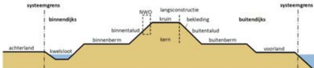
Figuur 2-1: Onderdelen van een dijk (BSD, WSRL 2017)
