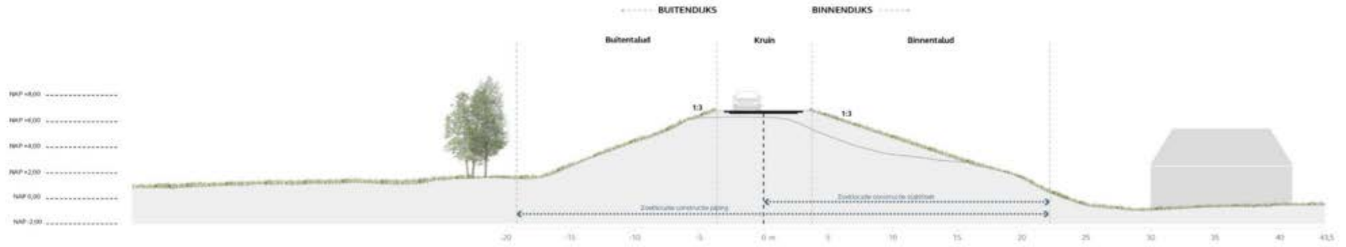
Dijkzone 10 – Vak 59 – Alternatief 1 en Alternatief 2 - Vak 60 – Alternatief 1 – Binnenwaartse kruinophoging en en constructie stabiliteit en piping
