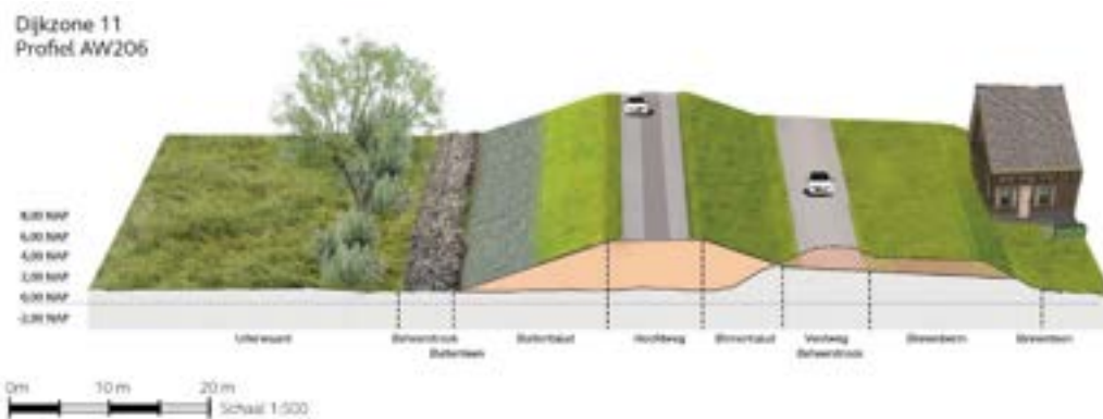
Figuur 14-13: Voorkeursalternatief dijkzone 11 3D-visualisatie (dijkvak 81, 82 en 86a)
