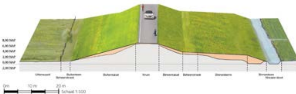
Figuur 8.10: Voorkeursalternatief dijkzone 4 3D-visualisatie dijkvak 27a en 27b
