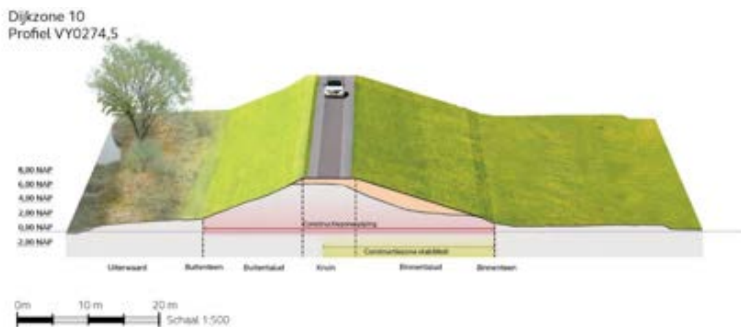
Figuur 13-5: Voorkeursalternatief dijkvak 59 3D-visualisatie voor constructie met binnenwaartse kruinverhoging
