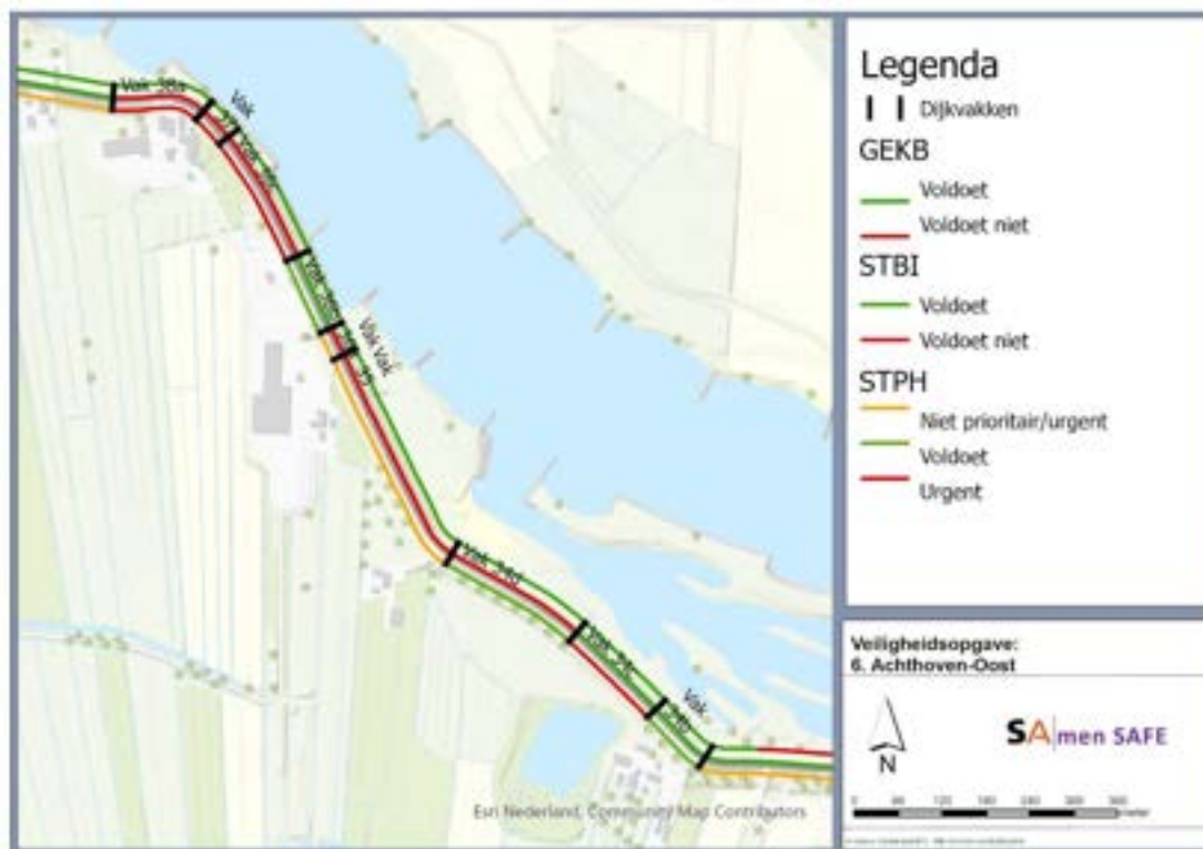
Figuur 9.2: Veiligheidsopgave planuitwerkingsfase dijkzone 6. De rode lijn geeft aan welke delen niet voldoen aan de
