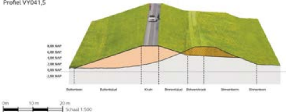
Figuur 8.9: Voorkeursalternatief dijkzone 4 3D-visualisatie dijkvak 26a
