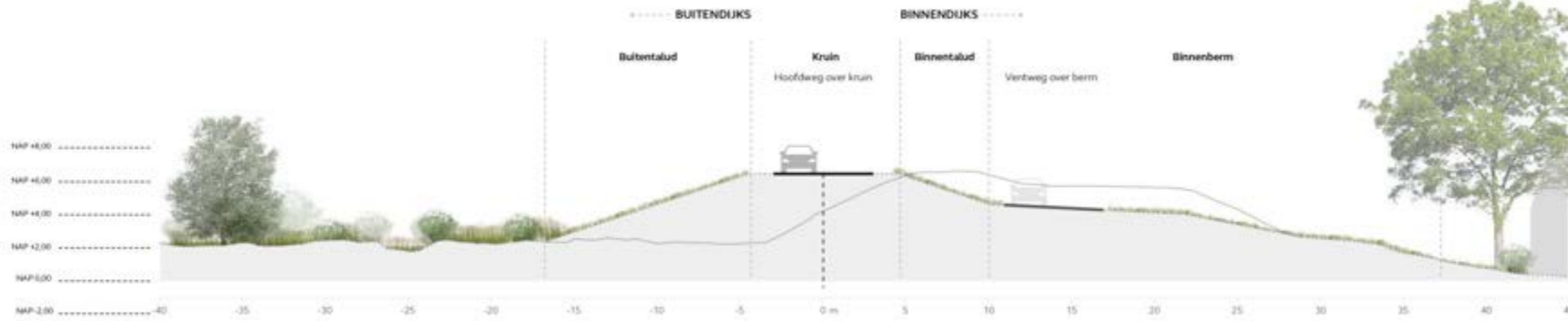
Dijkzone 11 – Vak 81+82+86a – Alternatief 1 – Buitenwaartse asverschuiving, kruin 9 m breed, hoofdweg op kruin en ventweg op berm
