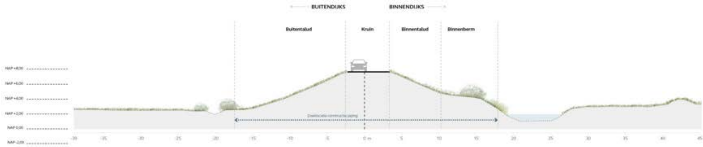
Dijkzone 2A – Vak 15+16a+17+18 – Alternatief 1 – Heavescherm
