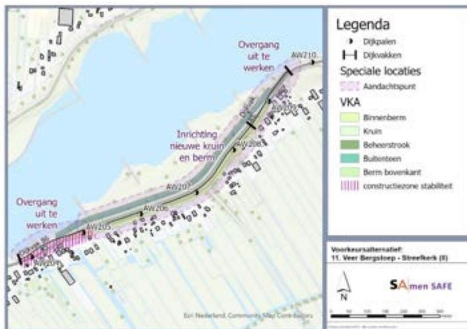
Figuur 14.2: Voorkeursalternatief dijkzone 11 dijkvakken 85 en 86 uit de verkenningsfase
